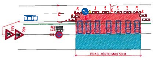
SCHEMA Č. 4 POSUVNÉ PRAC. MÍSTO V KOMUNIKACI + PARK. STÁNÍ A ZÁBOR CHODNÍKU
