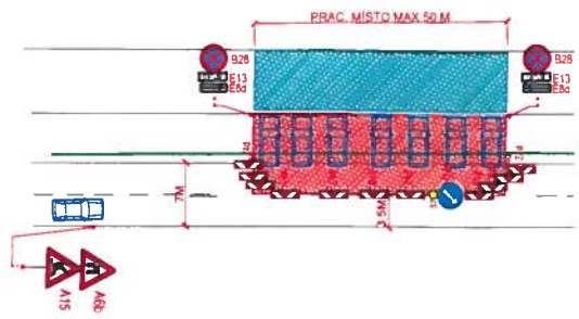
SCHEMA Č. 2 POSUVNÉ PRAC. MÍSTO V KOMUNIKACI + PARK. STÁNÍ A ZÁBOR CHODNÍKU
