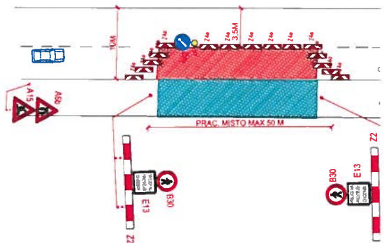
SCHEMA Č. 3 POSUVNÉ PRAC. MÍSTO V KOMUNIKACI UL. ČIHLÁŘSKÁ
